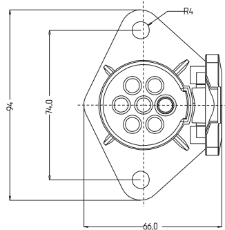
7'Lİ N TİPİ ALÜMİNYUM TIR RÖMORK FİŞİ (TERMİNALLI VE SOKETLİ) / 7 PIN ALUMINIUM TIR TRAILER PLUG (N TYPE)
