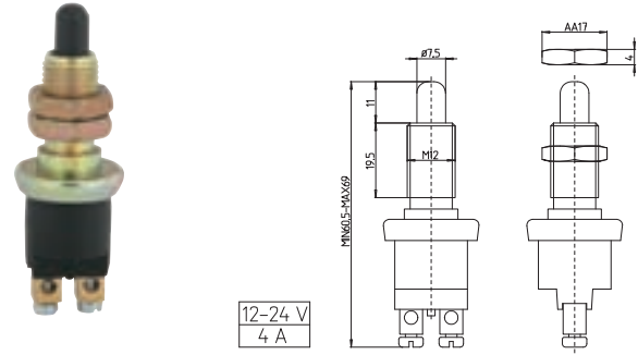
3600 FORD TRAKTÖR FREN OTOMATİĞİ 3600 FORD TRACTOR STOPLIGHT SWITCH
