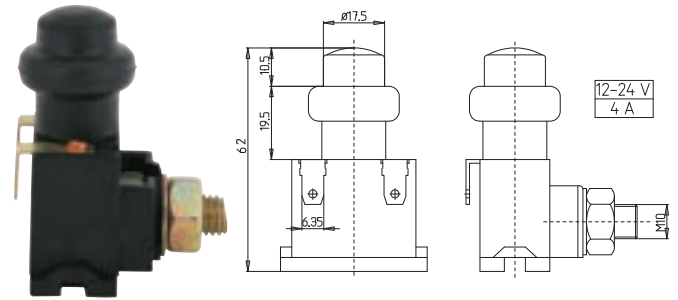
3600 FORD TRAKTÖR FREN OTOMATİĞİ 3600 FORD TRACTOR STOPLIGHT SWITCH
