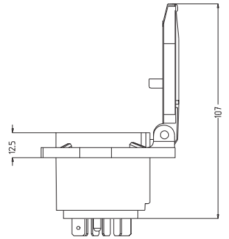
7'Lİ N TİPİ ALÜMİNYUM TIR RÖMORK FİŞİ (TERMİNALLI VE SOKETLİ) / 7 PIN ALUMINIUM TIR TRAILER PLUG (N TYPE)
