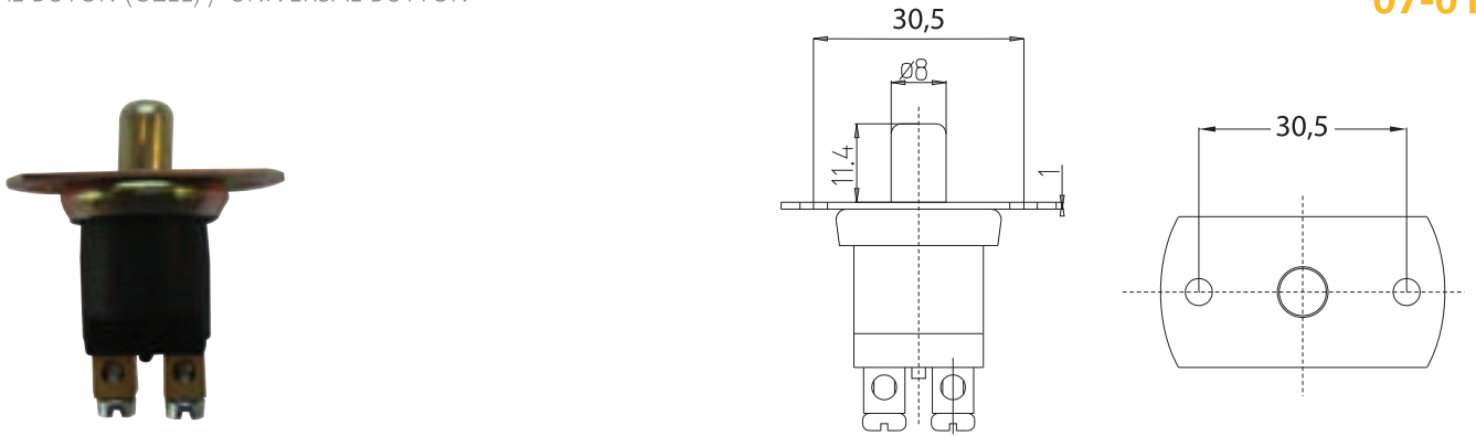
ÜNİVERSAL BUTON (ÖZEL) / UNIVERSAL BUTTON
