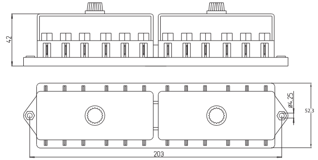
12'Lİ SİGORTA KUTUSU (BIÇAK SİGORTALI) / 12 WAY BLADE FUSE BOX WITH LUCAR TERMINALS
