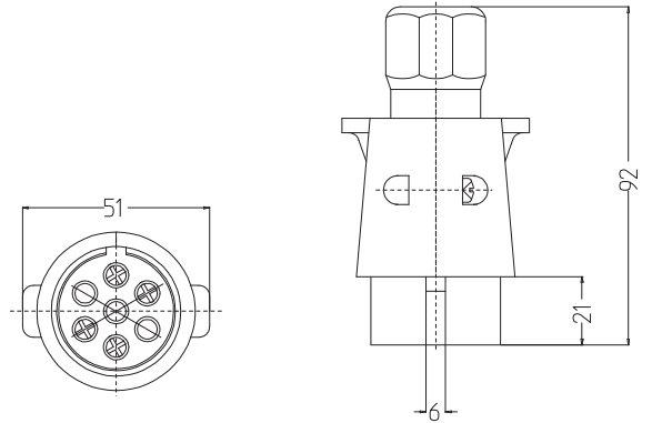
7'Lİ N TİPİ PLASTİK TRAKTÖR RÖMORK FİŞ VE PRİZ TAKIMI (VİDALI) / 7 PIN TRAILER PLUG & SOCKET (N TYPE)
