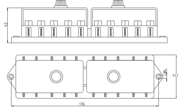
10'LU SİGORTA KUTUSU (BIÇAK SİGORTALI) / 10 WAY BLADE FUSE BOX WITH LUCAR TERMINALS
