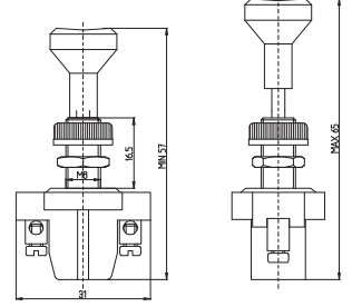
TEKLİ ÇEKME LAMBA ANAHTARI UZUN PASO LONG PUSH-PULL SWITCH
