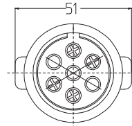
7'Lİ S TİPİ PLASTİK TRAKTÖR RÖMORK FİŞ VE PRİZ TAKIMI (VİDALI) / 7 PIN TRAILER PLUG & SOCKET (S TYPE)
