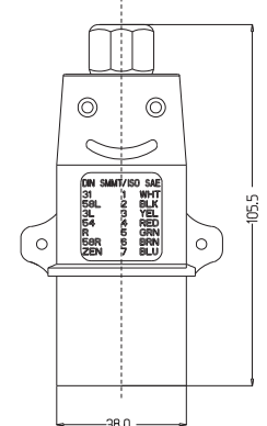
7'Lİ N TİPİ ALÜMİNYUM TIR RÖMORK FİŞİ (TERMİNALLI VE SOKETLİ) / 7 PIN ALUMINIUM TIR TRAILER PLUG (N TYPE)
