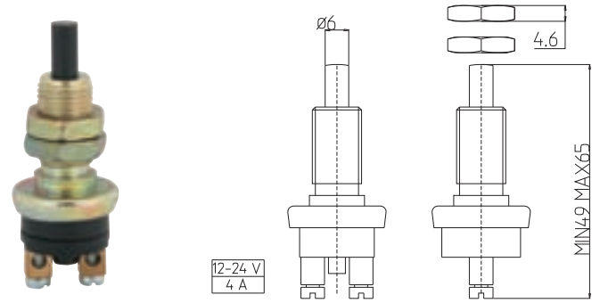
TRAKTÖR FREN OTOMATİĞİ (SIZDIRMAZLIK ÖZELLİĞİNE SAHİPTİR) BRAKE LIGHT SWITCH FOR TRACTOR AND H/D MACHINERY (IMPERMELABILITY)
