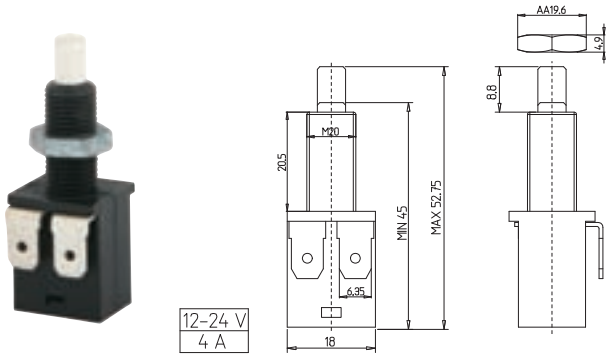
5000 FORD TRAKTÖR FREN OTOMATİĞİ (METAL) 5000 FORD TRACTOR STOPLIGHT SWITCH (METAL)
