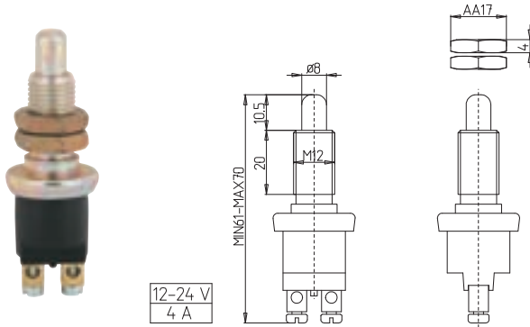
5000 FORD TRAKTÖR FREN OTOMATİĞİ (METAL) 5000 FORD TRACTOR STOPLIGHT SWITCH (METAL)
