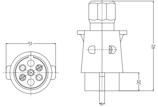
5'Lİ N TİPİ PLASTİK TRAKTÖR RÖMORK FİŞ VE PRİZ TAKIMI (VİDALI) / 5 PIN TRAILER PLUG & SOCKET (N TYPE)
