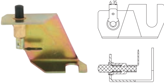
FIAT FREN OTOMATİĞİ (METAL GÖVDE-PLASTİK MİL GÜMÜŞ KONTAKLI) FIAT BRAKELIGHT SWITCH (WITH SILVER CONTACT)
