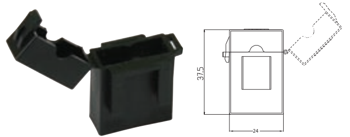
MAXİ SİGORTA KUTUSU BIÇAK TİPİ SİGORTA İÇİN MAXI FUSE HOLDER BLADE TYPE 01-018
