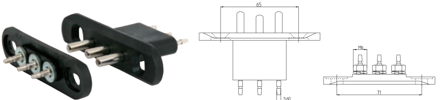
KAPI BUTONU (PANELVAN SÜRGÜLÜ KAPILAR İÇİN - ÜÇ FİŞLİ) / PANELVAN SLIDING DOOR BUTTON
