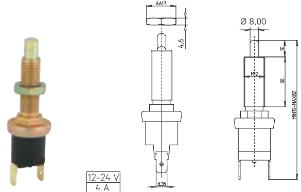
FIAT FREN OTOMATİĞİ (METAL) FIAT STOPLIGHT SWITCH (METAL)
