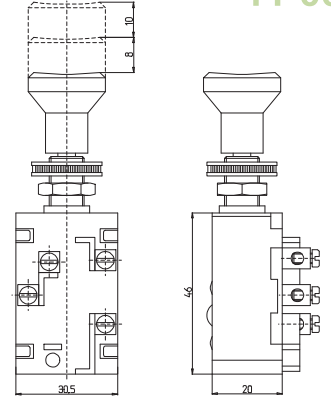
TEKLİ ÇEKME LAMBA ANAHTARI UZUN PASO LONG PUSH-PULL SWITCH
