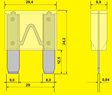
MAXI BIÇAK SİĞORTA MAXI BLADE FUSE
