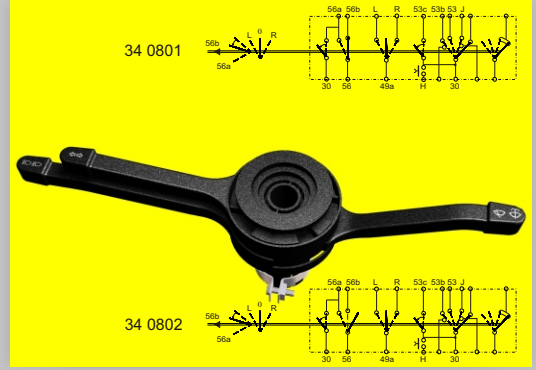
34 0801 TOFAŞ 131 SİNYAL KOLU Y.M. 34 0802 TOFAŞ 131 SİNYAL KOLU E.M. 34 0804 SERÇE SİNYAL KOLU STEERING COLUMN SWITCH
