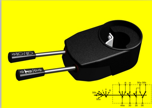
34 0512 50 NC SINYAL KOLU
