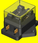
26 0200 YM. SİGORTA KUTUSU (2'Li)
