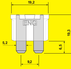
BIÇAK SİĞORTA BLADE FUSE
