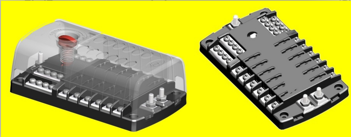
26 0500 12'Lİ SİGORTA KUTUSU NEGATİF DAĞITIMLI (KAPAKLI)
