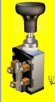
01 0502 ÇİFT ÇEKME Lİ ANAHTAR 20 A SİGORTALI
