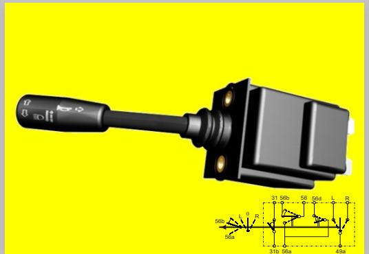
34 0530 TRAKTÖR SİNYAL KOLU STEERING COLUMN SWITCH
