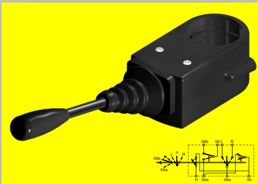
34 0524 STAYR SİNYAL KOLU
